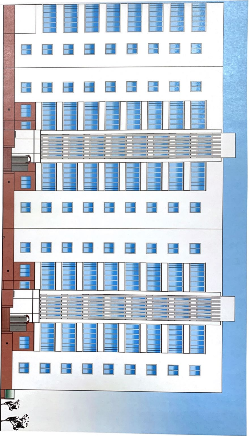
Фасад по оси 2 в осях Б - Г
